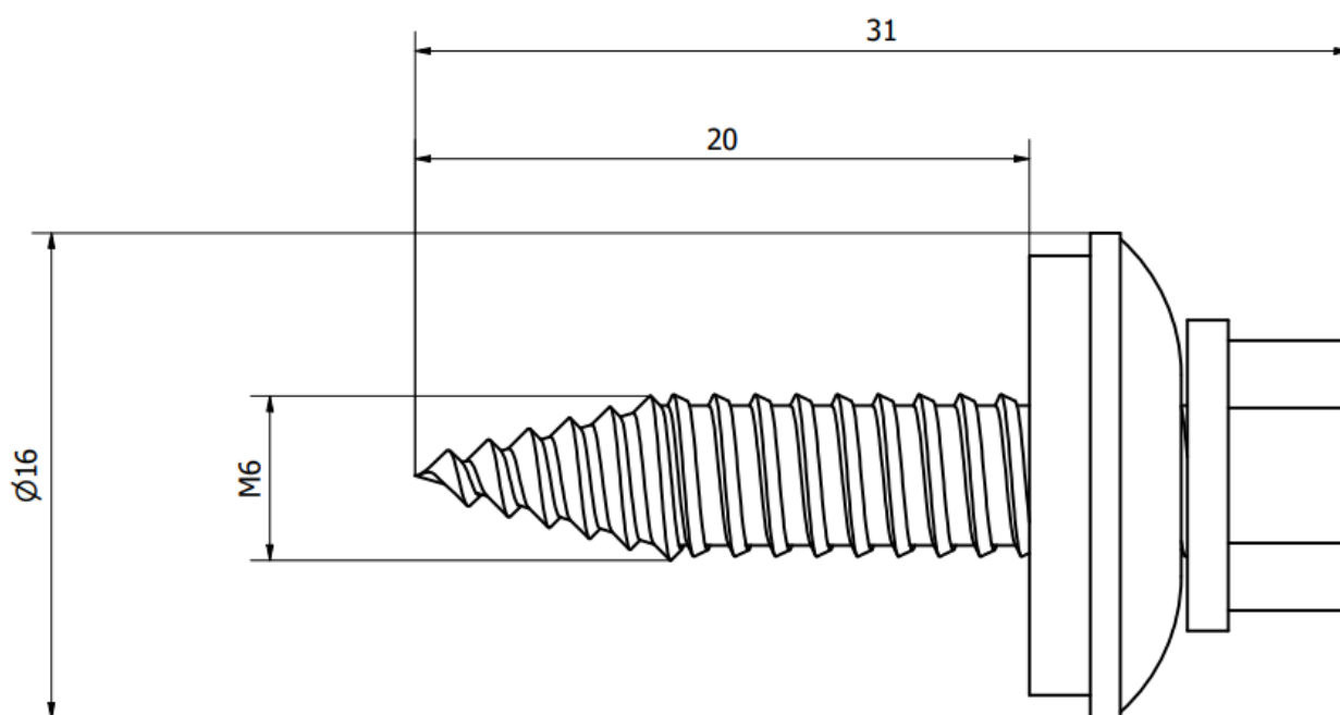
Rys.1 K-20 element dimensions
