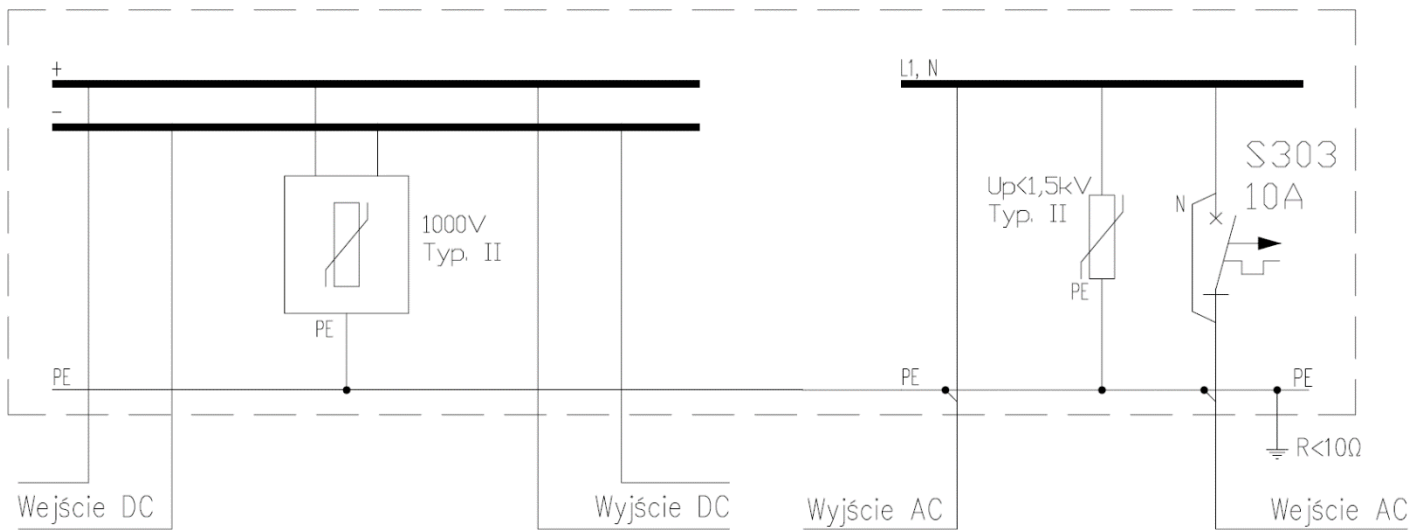
Rys.1. Schemat elektryczny rozdzielnic SOL-609
