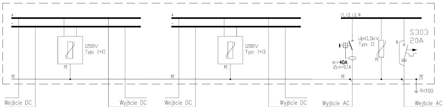
Rys.1. Schemat elektryczny rozdzielnic SOL-829
