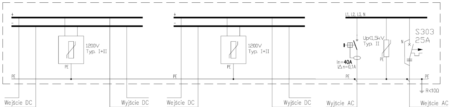
Rys.1. Schemat elektryczny rozdzielnic SOL-830
