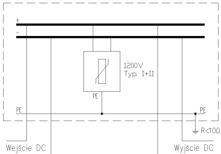
Rys.1. Schemat elektryczny rozdzielnic SOL-101
