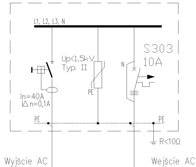
Rys.1. Schemat elektryczny rozdzielnicy SOL-515
