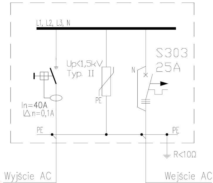
Rys.1. Schemat elektryczny rozdzielnic SOL-518
