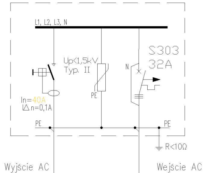
Rys.1. Schemat elektryczny rozdzielnic SOL-519
