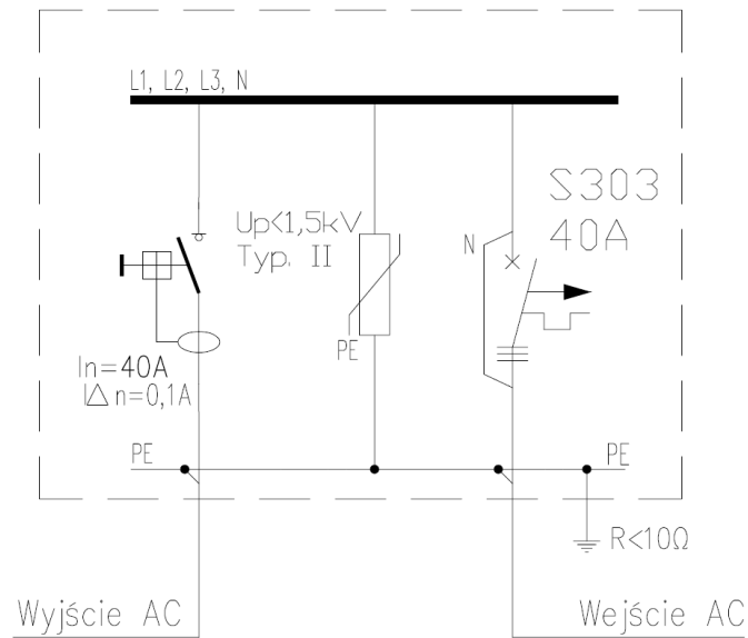
Rys.1. Schemat elektryczny rozdzielnic SOL-520
