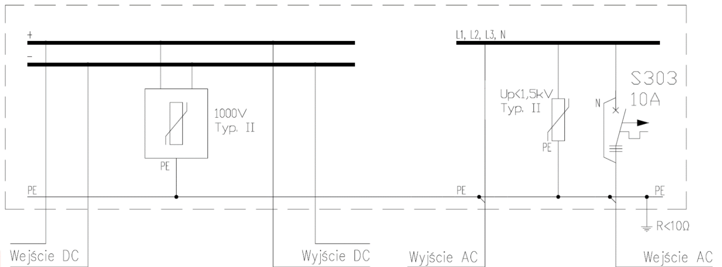
Rys.1. Schemat elektryczny rozdzielnic SOL-612
