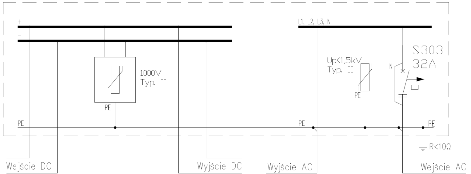
Rys.1. Schemat elektryczny rozdzielnic SOL-616
