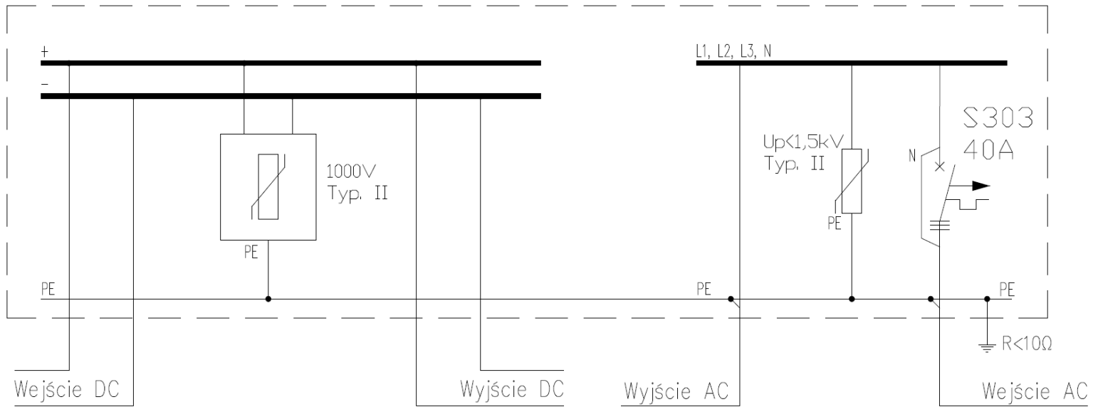
Rys.1. Schemat elektryczny rozdzielnic SOL-617
