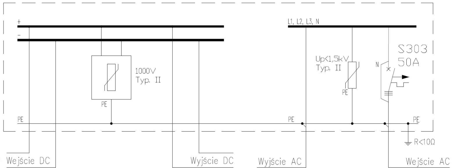
Rys.1. Schemat elektryczny rozdzielnic SOL-618
